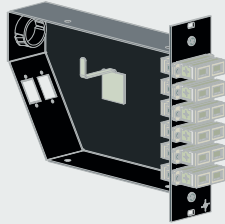
FanOut Module für TICNET-Strecke mit Kabelaufteiler Mini-ODS
